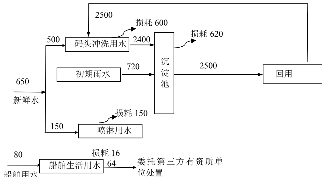
图 4-2 本项目水量平衡图 单位：t/a
