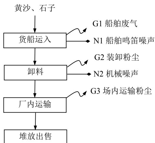
图 4-1 泊位装卸工艺流程及产污环节图
