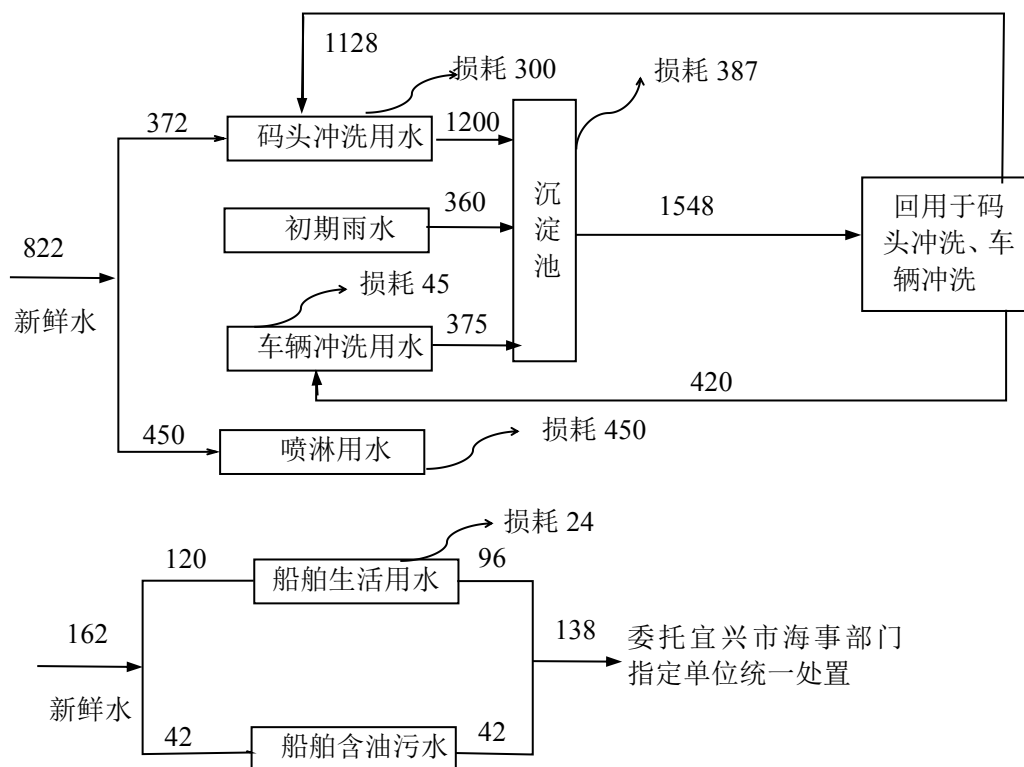
图 4-2 本项目水量平衡图 单位：t/a
