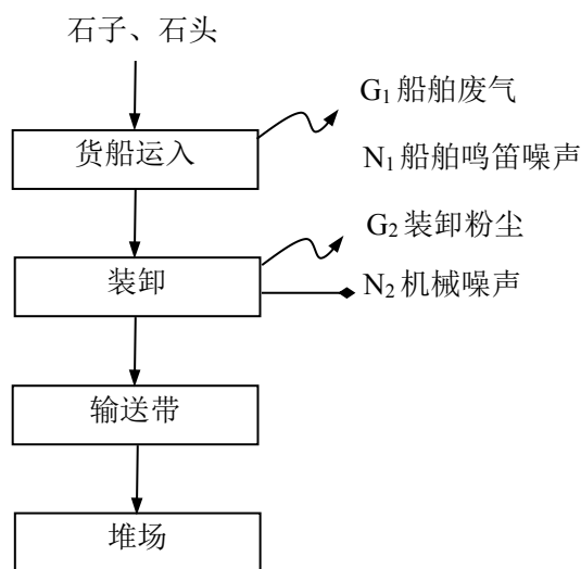
图 2.1-1 码头装卸工艺流程及产污环节图
