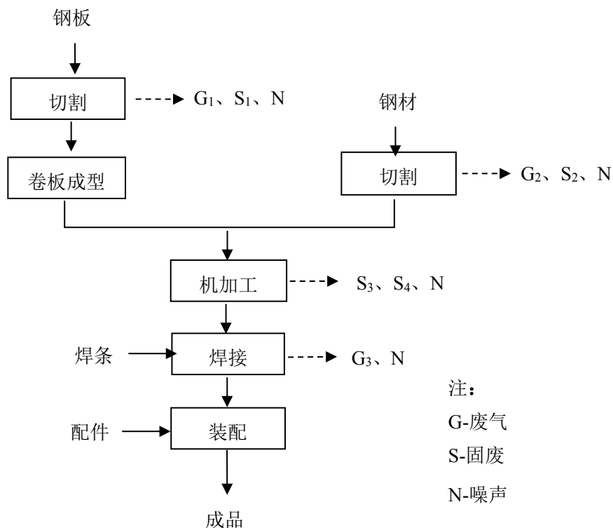
图 5-1 环保设备生产工艺流程及产污环节图
